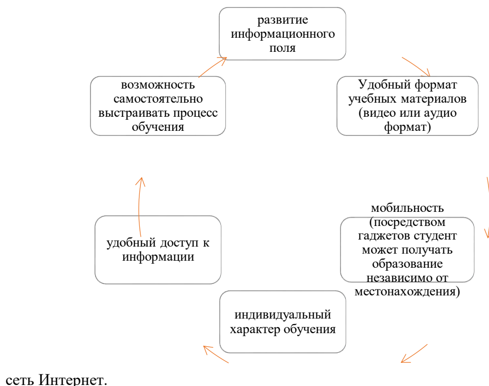
Рис. 8. Преимущества ЦОС
